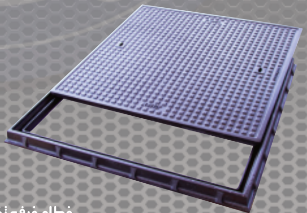
غطاء غرف نفيش ١٠٠ × ١٠٠ مع حمل اختبار ٤٠ / ٢٥ / ١٢,٥ / ١,٥ طن
