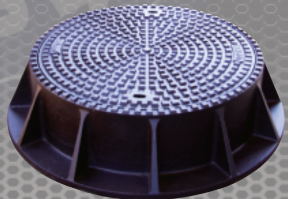
غطاء صرف صحي قطر داخلي ٦٠٠ مم وزن ٢٨٥ كغ من الزهر الرمادي
