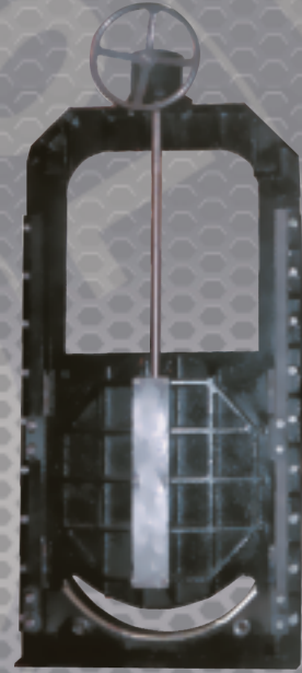
بوابة بجسج معلق غير طاعمة زهر مرن / زهر رمادي مقاسات مختلفة
