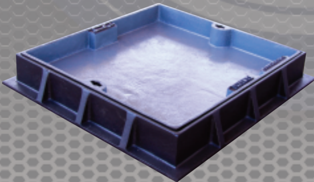
غطاء غرفه نفيش للخرسانة و الإنترنت مقاس داخلى ٦٠ × ٦٠ سم عمق ٧ سم حمل اختبار ٢٥ / ٤٠ طن
