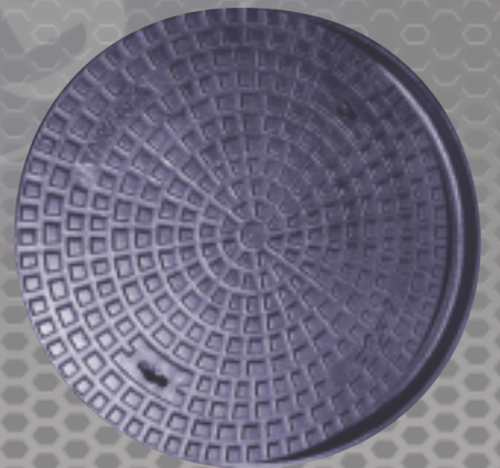
غطاء صرفه صدى من الزهر الرمادى قطر داخلى ٥٠٠ / ٦٠٠ مع حمل إختبار ١,٥ - ١٢,٥ طن
