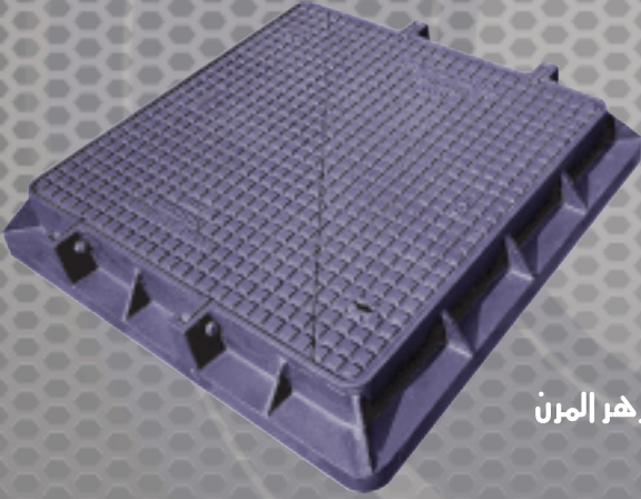
غطاء صرفه صدى قطر داخلى ٨٠٠ مع بمفصلة حمل إختبار ٤٠ طن من الزهر المرن
