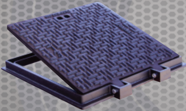
غطاء غرفه نفثيش موديل حرفه T بمفطلائه مقاس داخلى 60 × 60 / 50 × 50 / 40 × 40 حمل إختبار 1,5 / 12,5 / 20 / 40 طن من الزهر المرن
