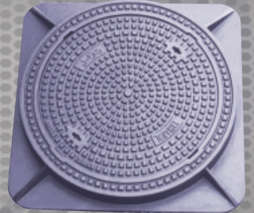
غطاء زهر رمادى قطر داخلى ٦٠٠ مع حمل إختبار ٢٥ - ٤٠ طن القاعدة مربعة من أسفل و بحلية دائرية علوية
