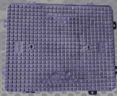
غطاء غرف التفتيش للمحابس من الزهر المرن مقاس داخلي ٧٥٠ × ٦٠٠ مع حمل اختبار ٢٥ / ١٢,٥ طن
