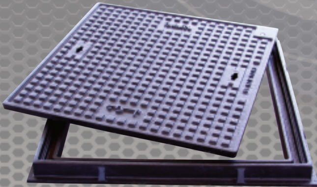
غطاء غرفه نفثيش موديل الجزيرة مقاس داخلى 60 × 60 / 50 × 50 / 40 × 40 حمل إختبار 1,5 / 12,5 طن من الزهر الرمادى
