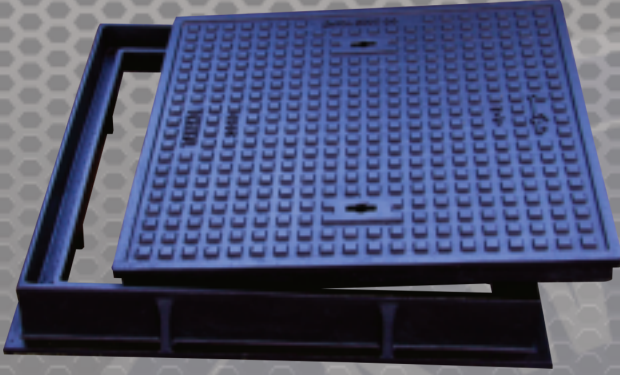
غطاء غرفه نفثيش 60 × 60 مع سنجل سيل حمل إختبار 20 / 40 طن
