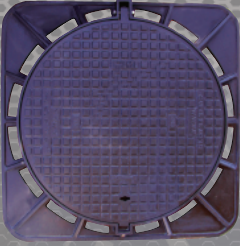
غطاء صرفه صدى قطر داخلى ٨٠٠ مع بمفصلة حمل إختبار ٤٠ طن من الزهر المرن
