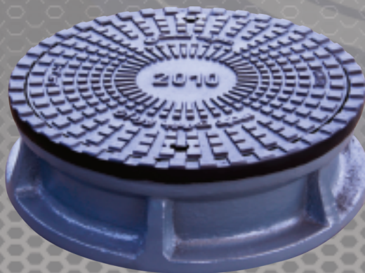
غطاء صرف صحي موديل الهيئة قطر ٦٠٠ مم قطر داخلي ٥٣٠ مم وزن ٢٨٥ كغ من الزهر الرمادي
