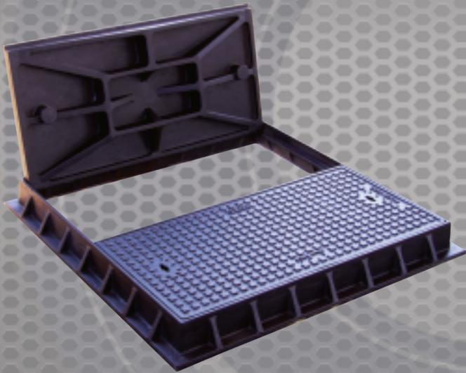
غطاء غرف نفيش مقاس داخلية ٦٠ × ٩٠ مع حمل اختبار ٤٠ / ٢٥ / ١٢,٥ طن
