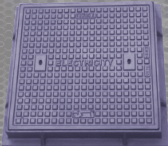
غطاء غرف نفثيش كهرباء - تليفونات مقاس داخلى ٤٠٠ × ٤٠٠ / ٦٠٠ × ٦٠٠ / ٩٠٠ × ٩٠٠ مع حمل إختبار ٢٥ / ٤٠ طن من الزهر المرن
