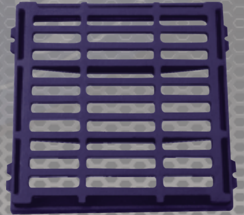
غطاء صرف مياه الأمطار ٢ قطعة مقاس ٥٠٠ × ٥٠٠ مع حمل إختبار ٢٥ طن من الزهر المرن
