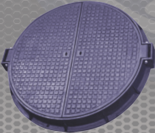
غطاء غرفه تفنيش المحابس من الزهر المرن قطر داخلى ١٢٥٠ مع ٢ طبة نصف دائرية بمفصلات حمل إختبار ٤٠ طن
