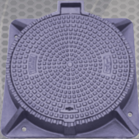
غطاء صرفه صدى القاهرة بمفصلة قطر داخلى ٦٠٠ مع حمل إختبار ٤٠ طن من الزهر الرمادى
