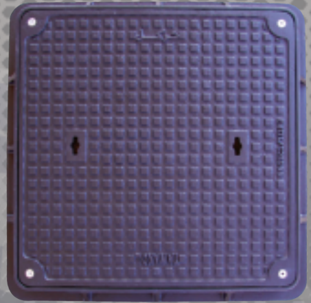
غطاء غرف نفيش مانع مياه مقاس داخلية ٥٠ × ٥٠ - ٦٠ × ٦٠ - ٨٠ × ٨٠ مع حمل اختبار ٤٠ / ٢٥ / ١٢,٥ / ١,٥ طن
